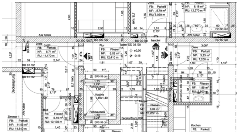
Planauszug Ausführungsplanung
